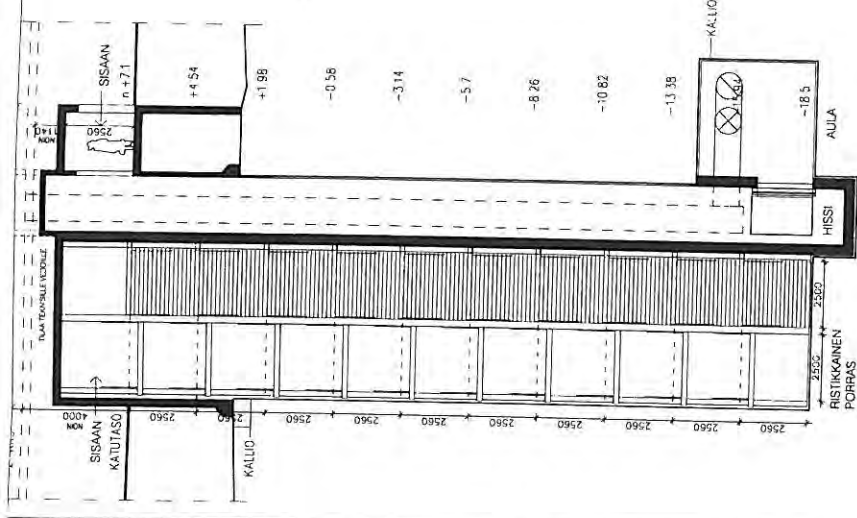
RISTIKÄINEN POKRAS B-B
